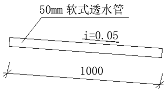
图C. 26 排水管大样图
