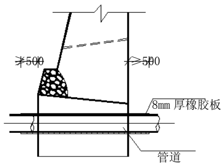
图C.4 挡土墙立面 1-1 剖面图
