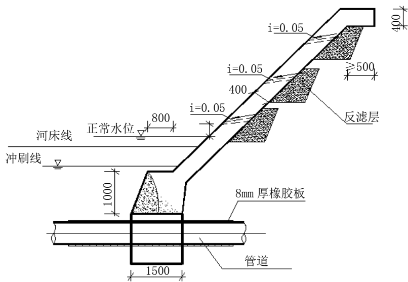
图C.7 坡式护岸立面 1-1 剖面图
