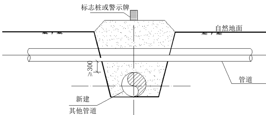
图A.10 新建其他管道穿越管道纵断面 A-A 剖视图
