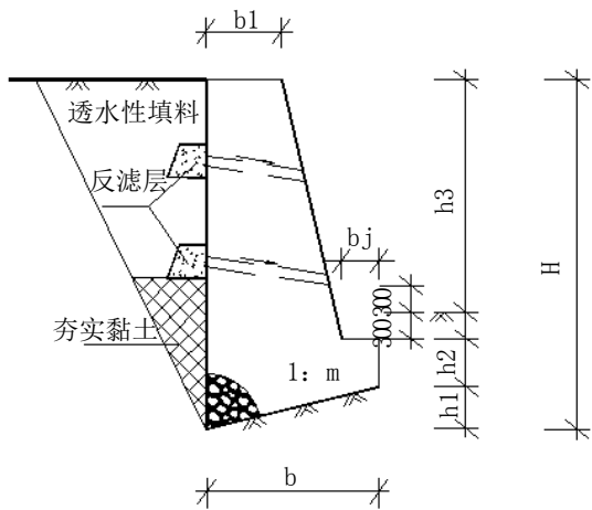
图C.2 挡土墙断面图
