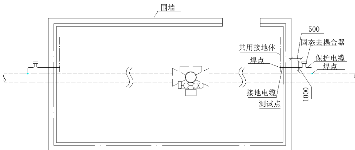
图B.7 工艺站场、监控阀室集中接地防护点安装图
