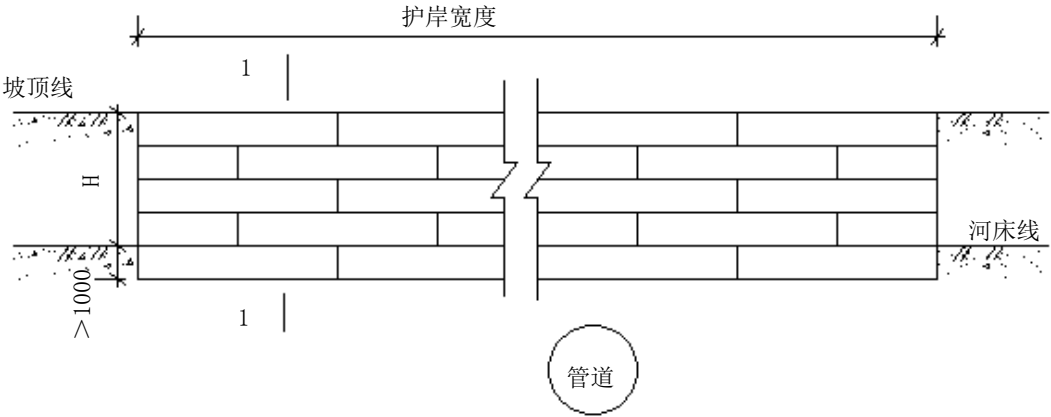
图C. 20 石笼护岸正立面图
