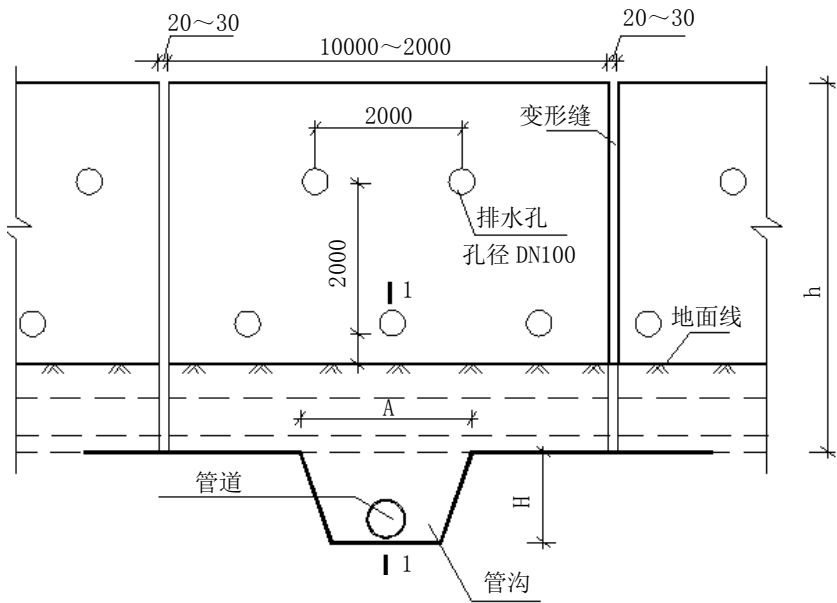
图C.1 挡土墙立面图
