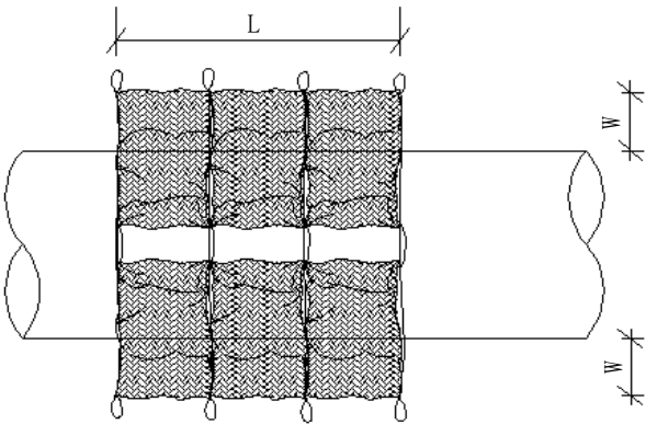
图C. 40 平衡压袋俯视图
