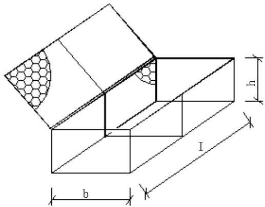
图C. 14 I 型石笼形式图
