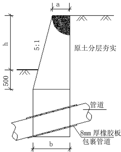
图C.31 堡坎立面图 1-1 剖面图
