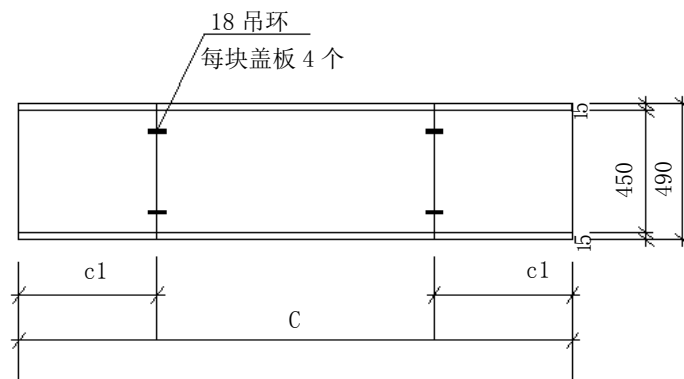
图A. 4 盖板吊环布置图
