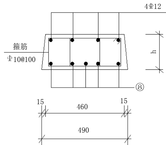
图A.5 盖板截面配筋图
