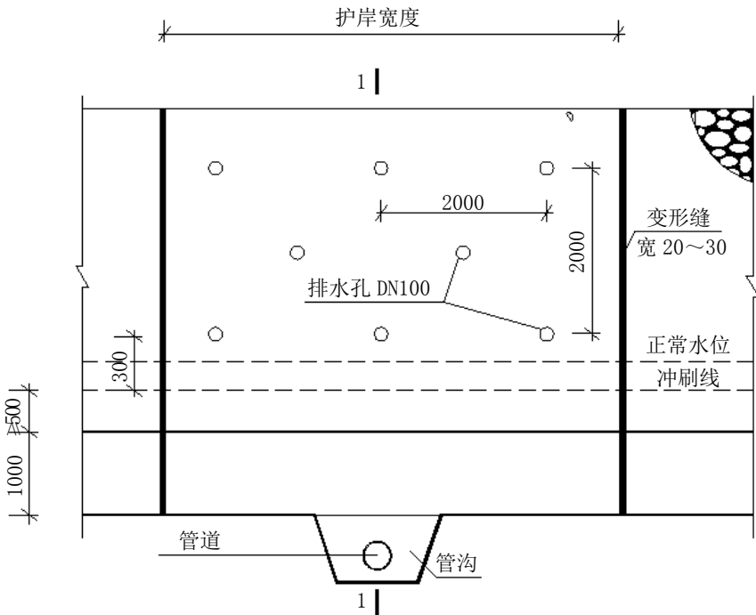
图C.6 坡式护岸立面图
