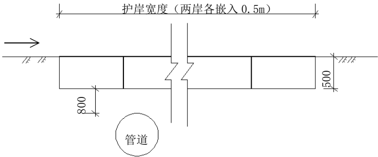
图C. 19 石笼护岸平面布置 1-1 剖面图
