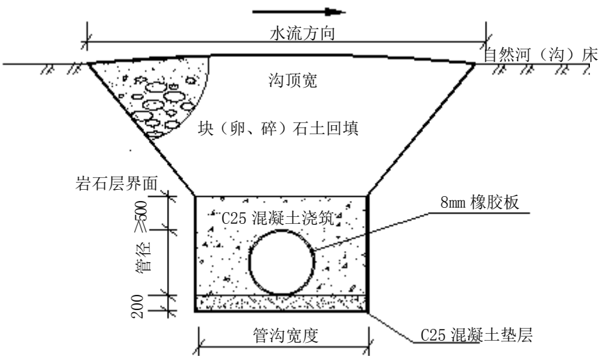
图C.13 A-A 断面示意图
