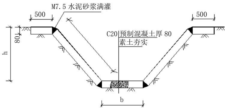
图C. 29 预制混凝土排水沟
