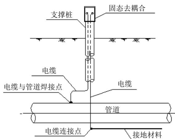
图B.2 交流干扰防护点接线图
