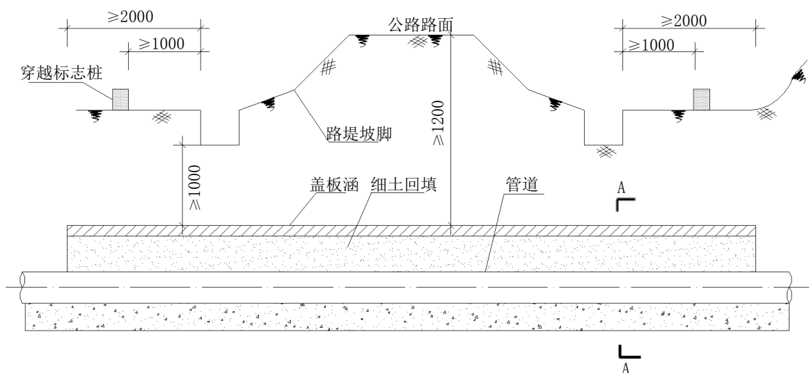
图A.1 新建公路采用盖板涵保护穿越管道纵断面图
