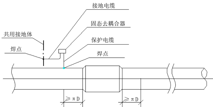
图B.8 监视阀室绝缘接头处集中接地防护点安装图
