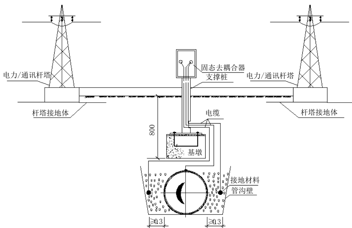
图B.6 强电冲击屏蔽防护安装图
