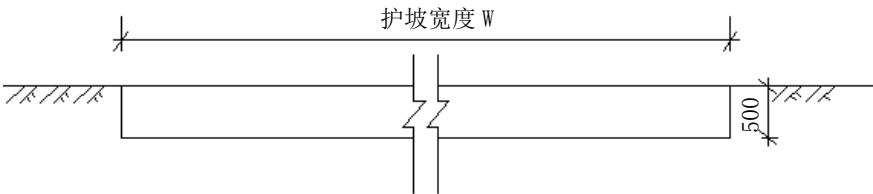
图C.34 草袋护坡正面 2-2 剖面图
