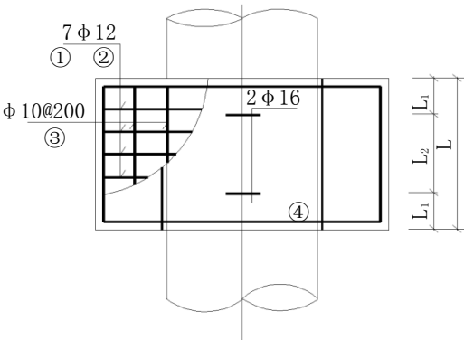
图C. 35 配重块平面图
