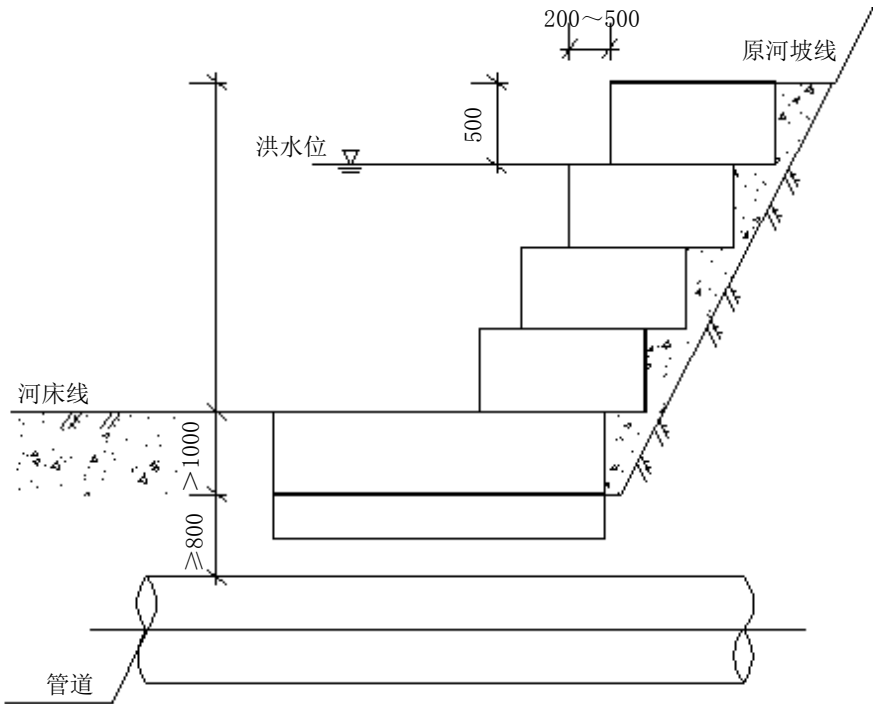
图C. 21 石笼护岸正立面 1-1 剖面图
