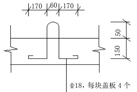
图A.6 盖板吊环详图
