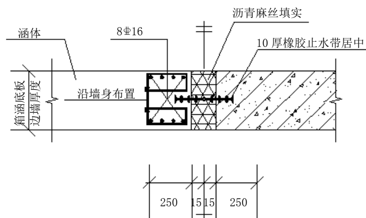
图A.7 变形缝详图
