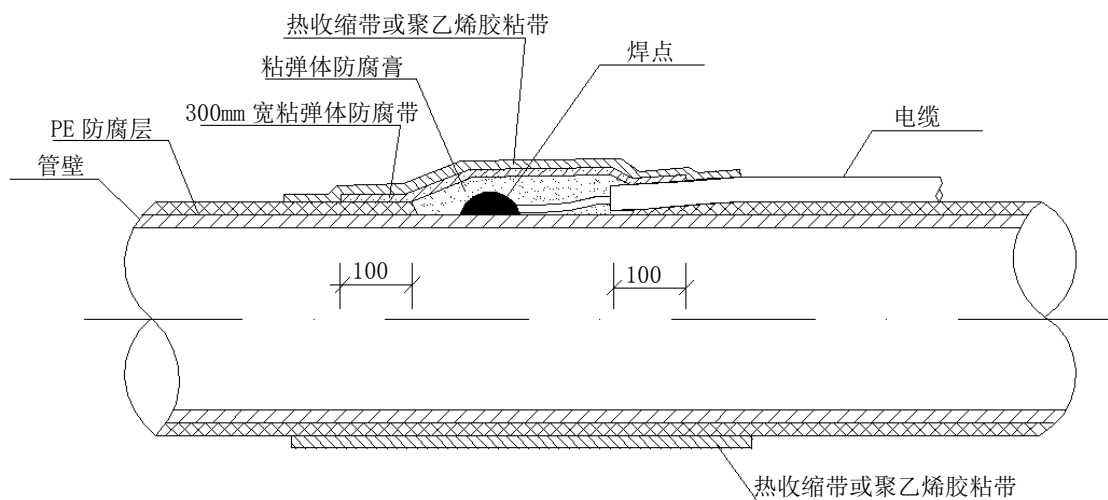
图B.11 电缆与管道焊接处防腐密封图
