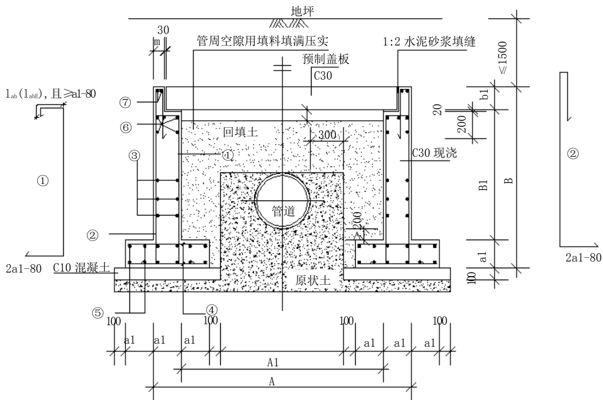
图A. 3 盖板涵详图
