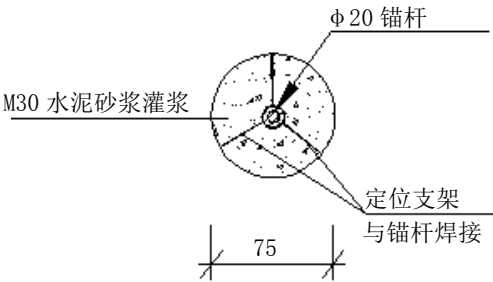
图C.27 锚杆横断面图
