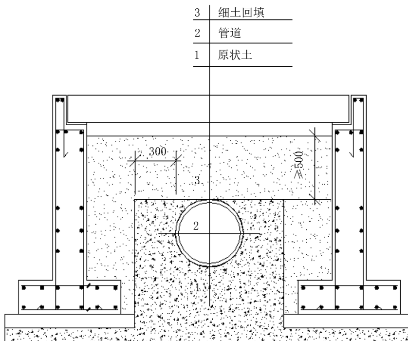
图A.2 盖板涵保护穿越管道纵断面 A-A 剖视图
