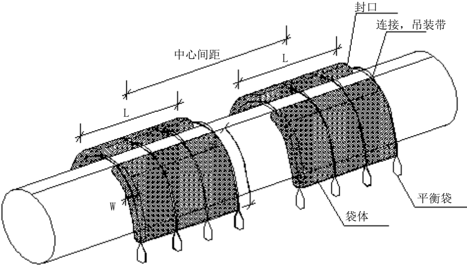
图C. 41 平衡压袋压载图
