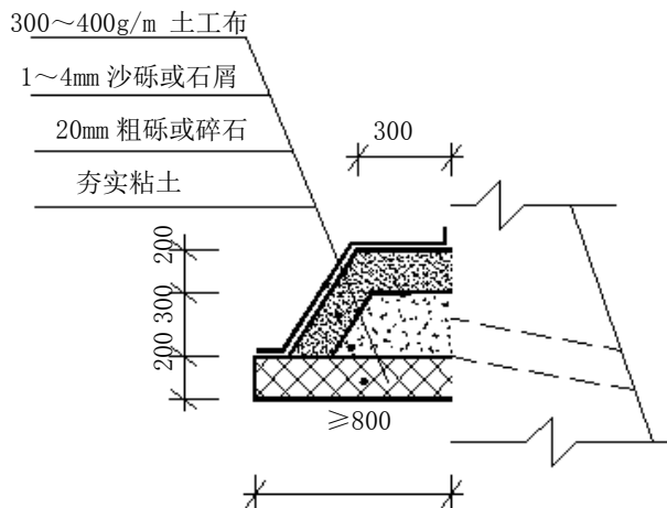
图C.3 反滤层大样
