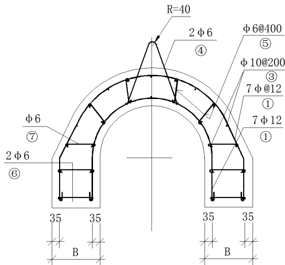
图C.37 配重块配筋图
