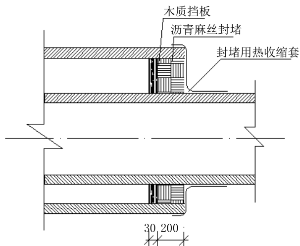
图A.15 封堵端封堵图
