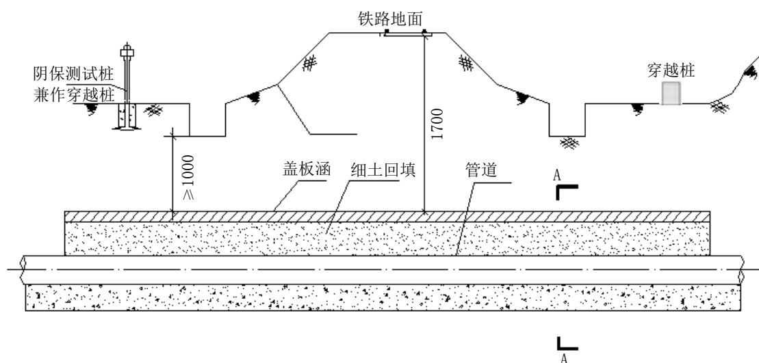
图A.8 新建铁路采用盖板涵保护穿越管道纵断面图
