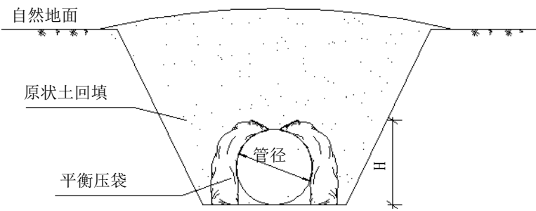
图C. 38 平衡压袋稳管断面图
