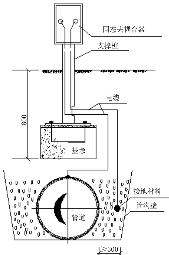
图B.1 交流干扰防护点测视图
