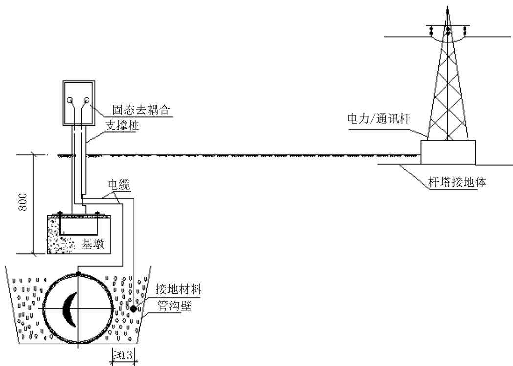
图B.4 强电冲击屏蔽防护安装图
