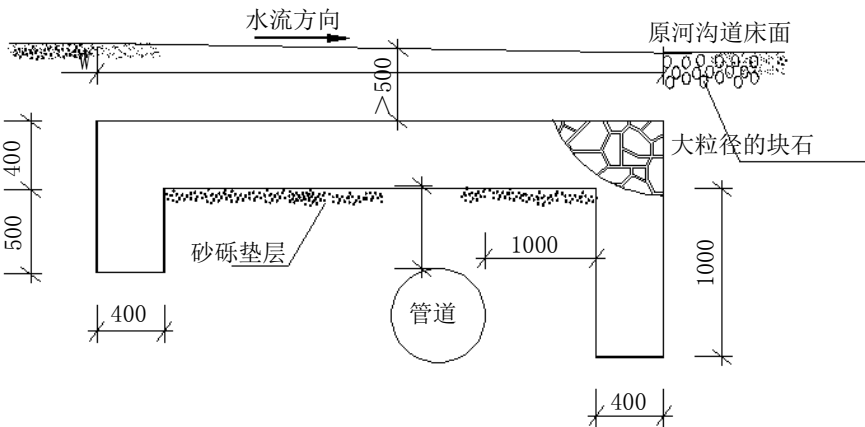
图C. 11 浆砌石过水面 1-1 剖面图
