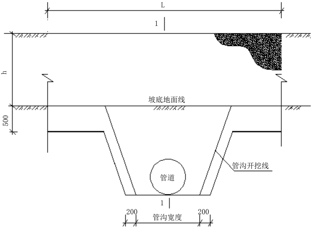
图C.30 堡坎立面图
