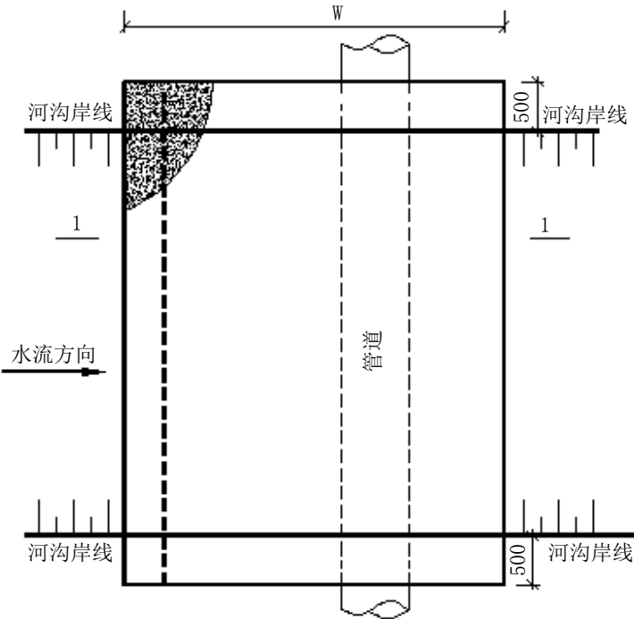
图C. 10 浆砌石过水面平面布置图
