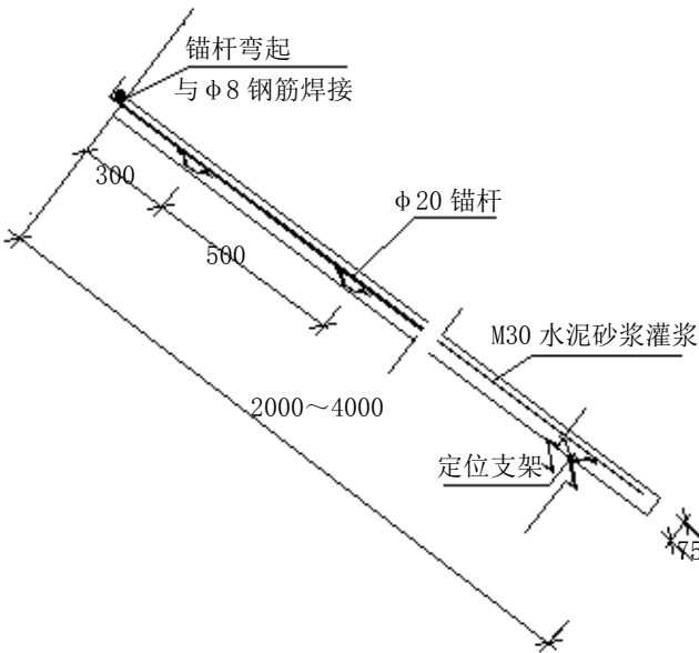
图C. 24 护面锚杆大样图
