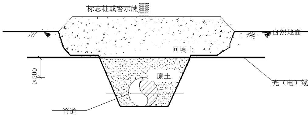
图A.12 电(光)缆穿越管道纵断面图 A-A 剖视图
