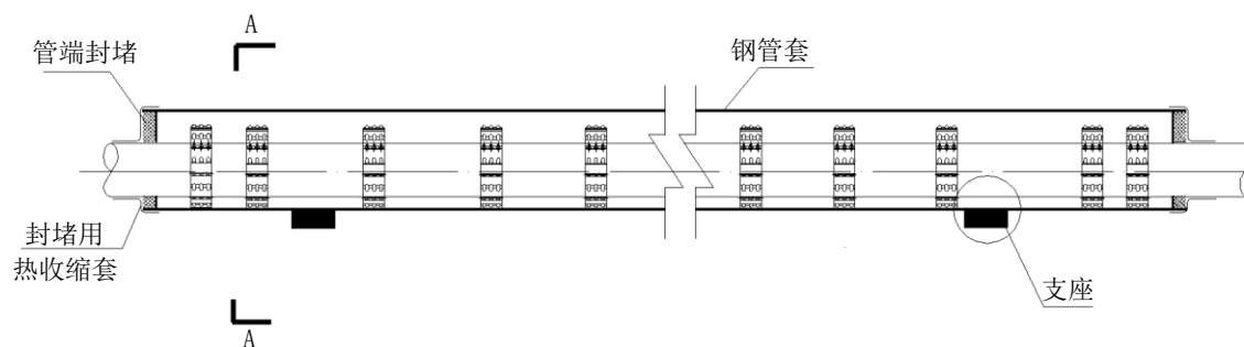
图A.13 钢套管保护纵断面示意图
