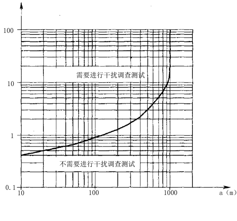
图 1 管道与 110kV 及以上高压交流输电线路的极限接近段长度 (L) 与间距 (a)
