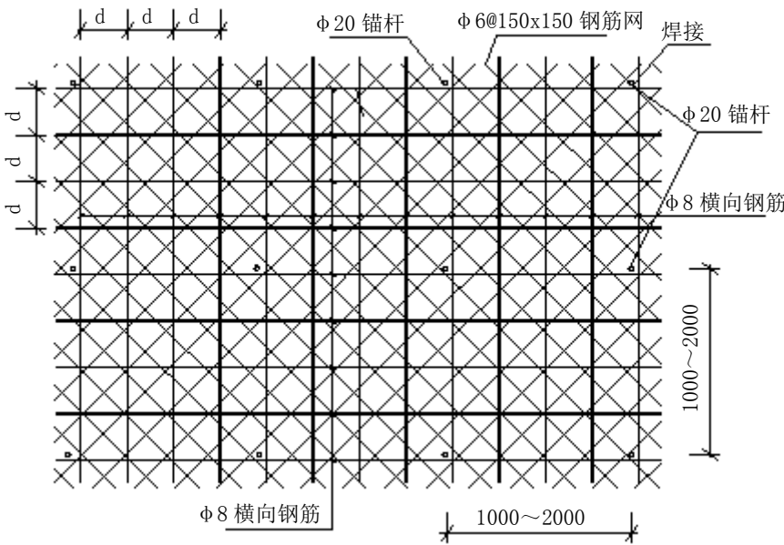
图C. 25 护面细部构造图
