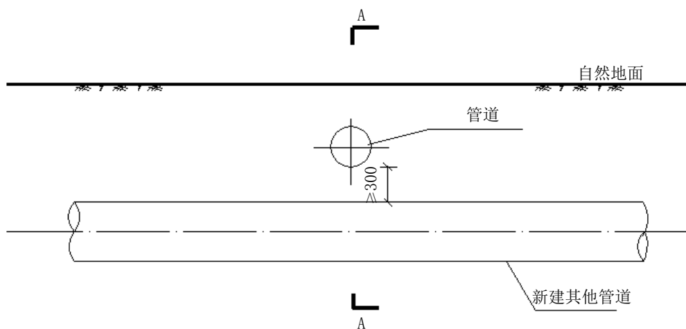
图A.9 新建其他管道穿越管道纵断面图
