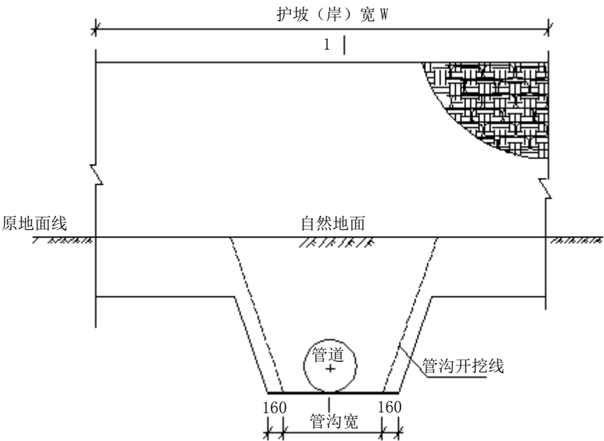
图C.32 草袋护坡正面图
