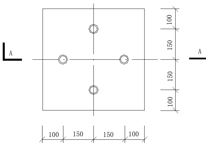
图B.13 基墩俯视图
