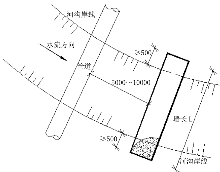
图C.8 地下防冲墙平面布置图
