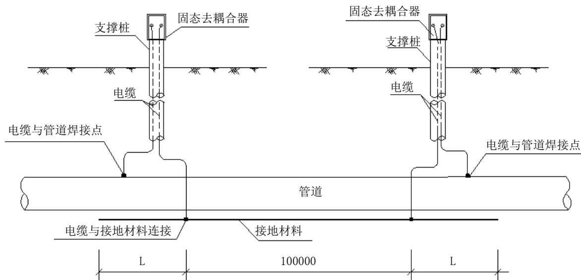
图B.3 强电冲击屏蔽防护接线图
