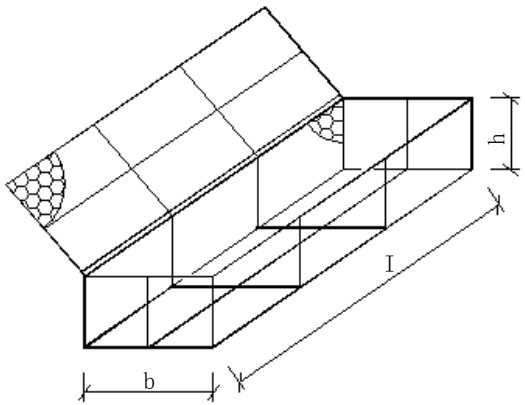
图C. 16 III 型石笼形式图
