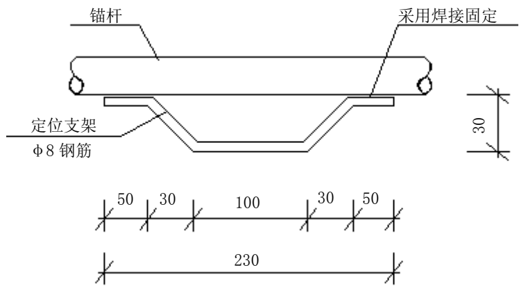
图C.23 护面锚杆定位支架
