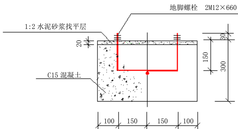
图B.14 基墩俯视 A-A 详图
