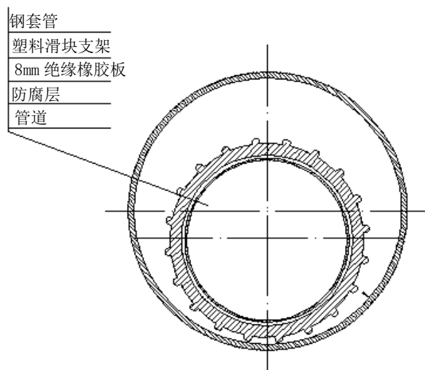
图A.14 钢套管保护纵断面示意图 A-A 剖面图
