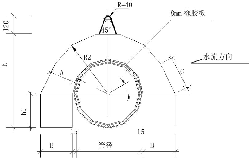
图C. 36 配重块立面图
