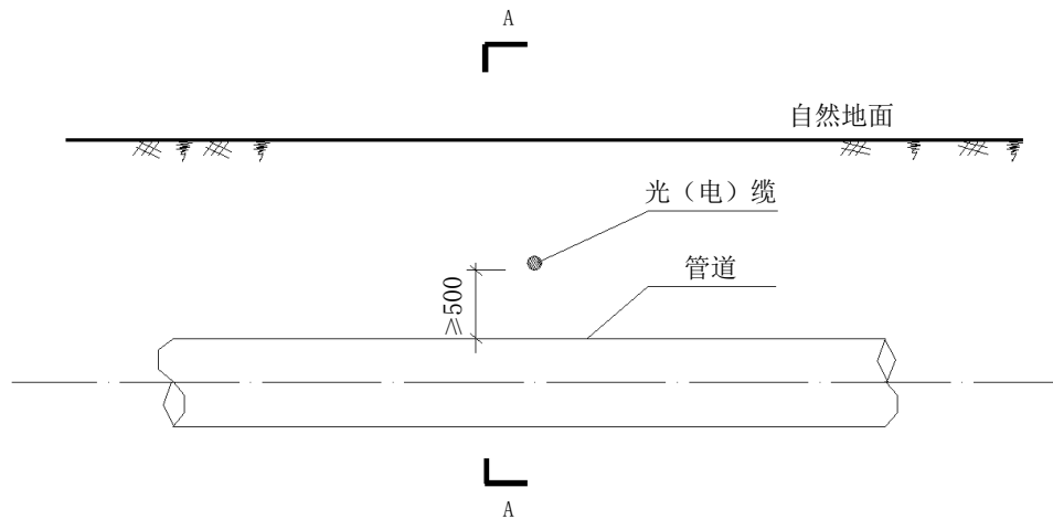
图A.11 电(光)缆穿越管道纵断面图
