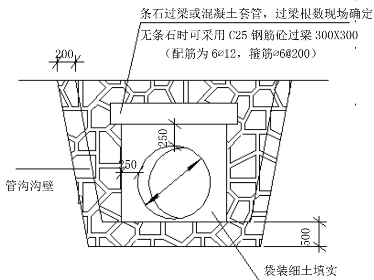
图C.5 挡土墙底管沟大样图
