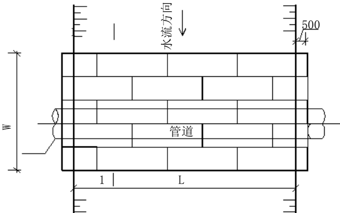
图C. 18 石笼护底平面布置图
