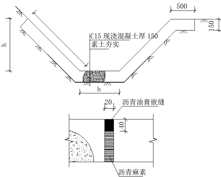
图C.28 现浇混凝土排水沟
