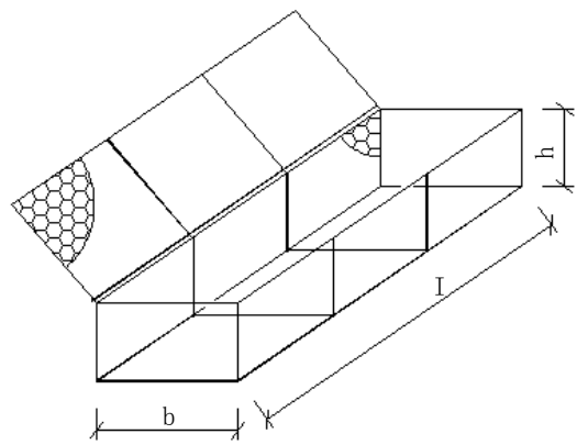
图C. 15 II 型石笼形式图
