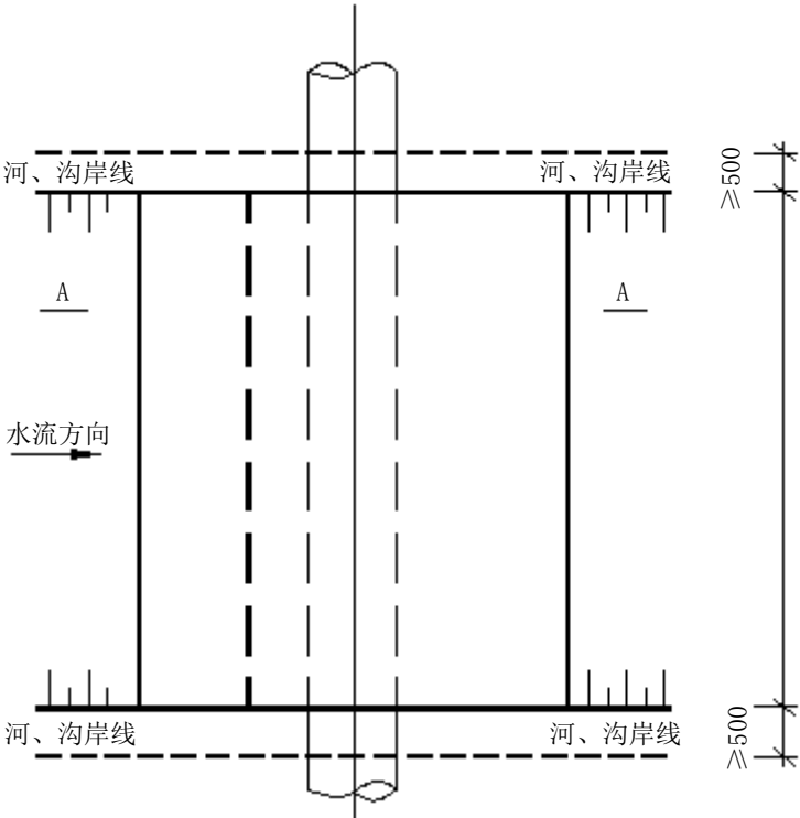
图C.12 混凝土连续覆盖平面图
