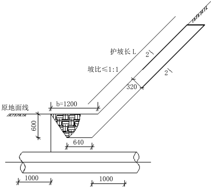
图C.33 草袋护坡正面 1-1 剖面图
