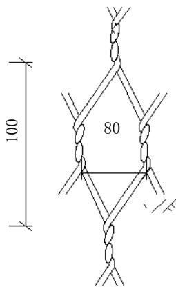
图C. 17 六角形铁丝石笼网孔图
