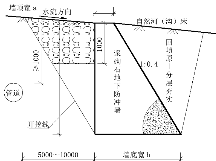
图C.9 地下防冲墙剖面图
