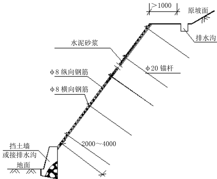
图C.22 护面剖面示意图
