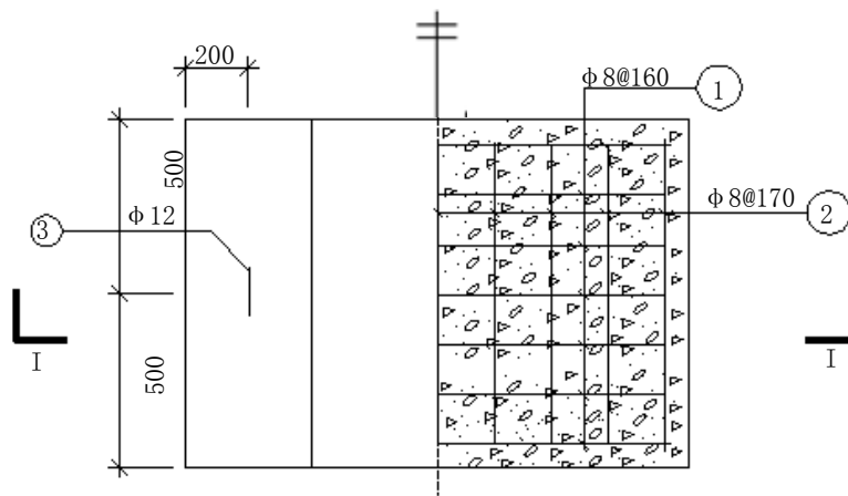
图A.16 支座板平面图
