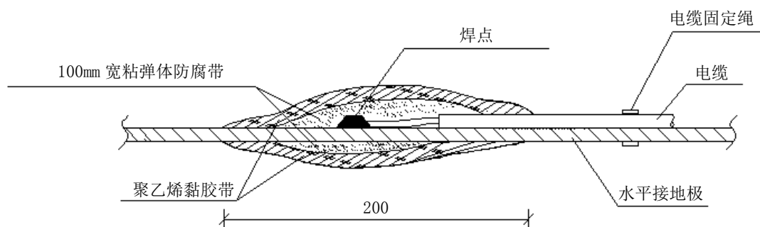
图B.12 电缆与接地极焊接点防腐密封图
